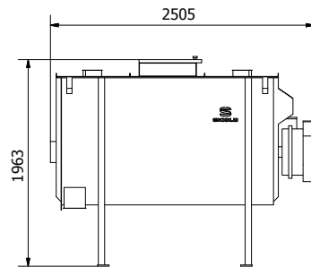
1-trins – kun blander
