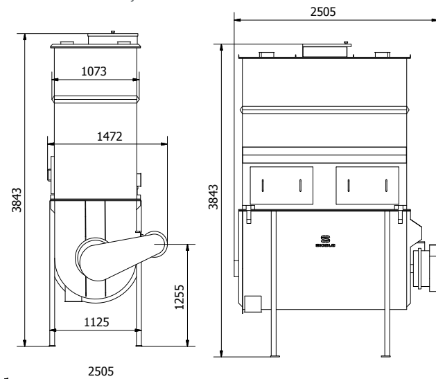
2-trins – blander + forbeholder + stativ
