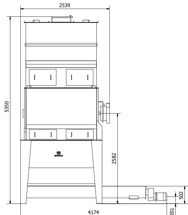
3-trins – blander + forbeholder + efterbeholder
