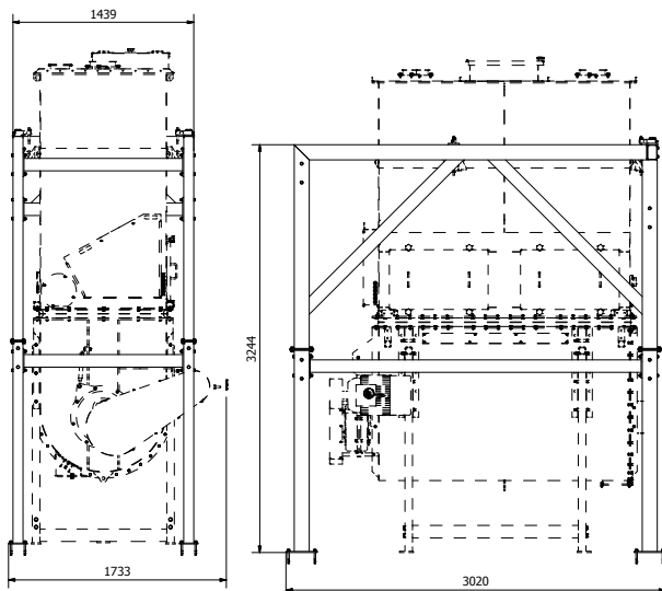
2-trins – blander + forbeholder + stativ
