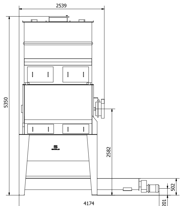
3-Stufen – Mischer + Vorbehälter + Entleerungsbehälter
