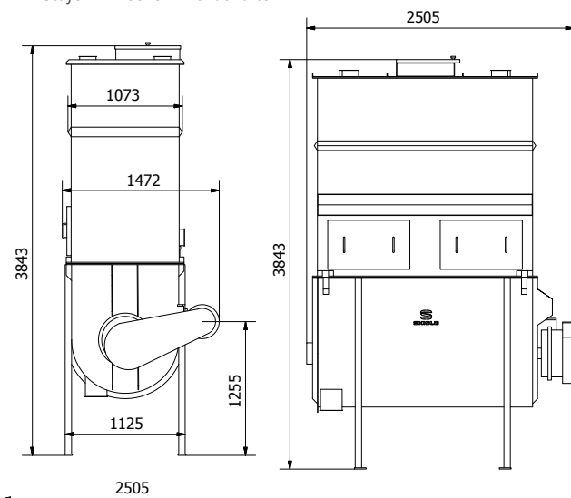
2-Stufen – Mischer + Vorbehälter + Gestell
