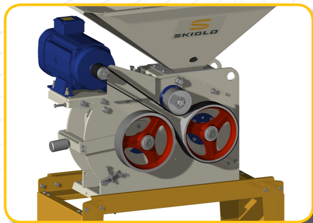
Poulie rainurée en fonte
